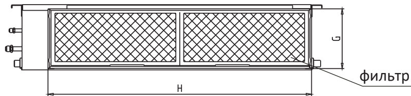
Сторона входа воздуха, размеры
