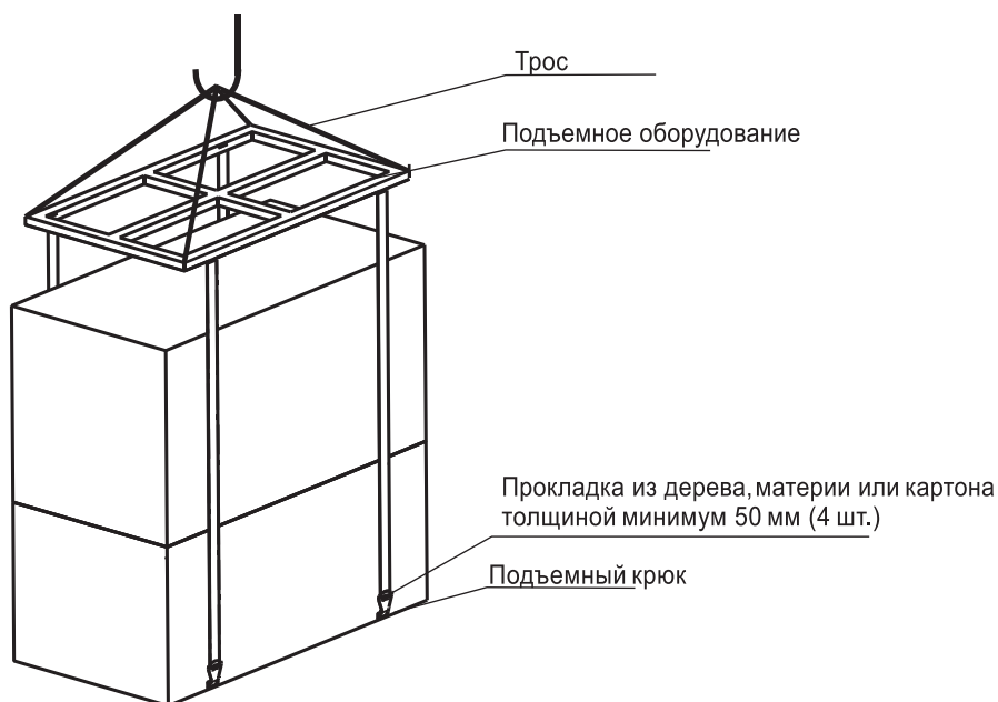
Рис. 5-1 Подъем установки
