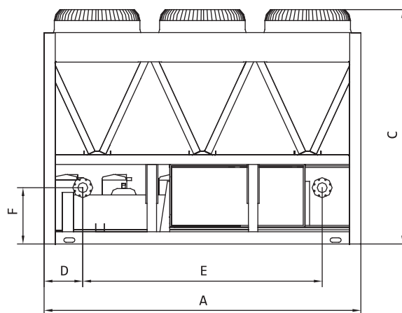
Вид спереди
