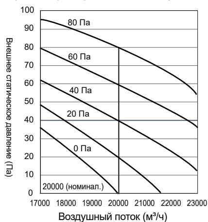
Кривая характеристик вентилятора 18 л. с.
