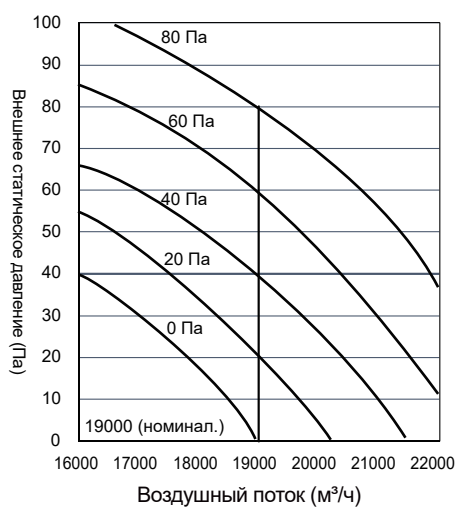
Кривая характеристик вентилятора 24 л. с.
