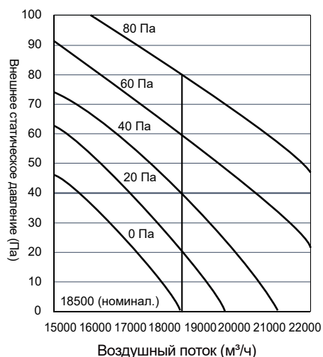
Кривая характеристик вентилятора 22 л. с.
