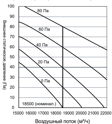
Кривая характеристик вентилятора 16 л. с.
