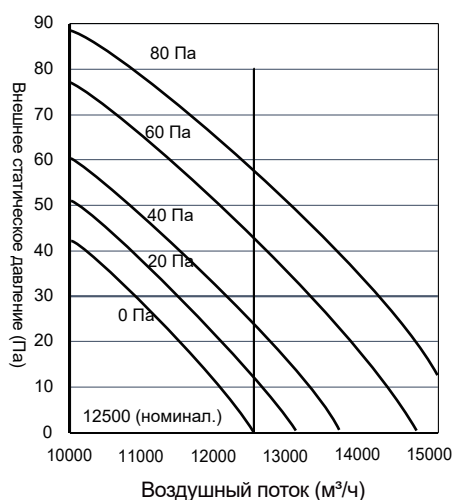
Кривая характеристик вентилятора 14 л. с.
