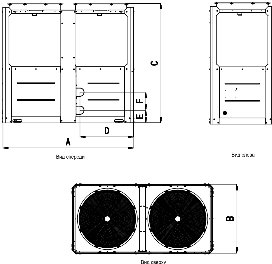
Габаритный чертеж для модели MDVM-V180D2BR8-A
