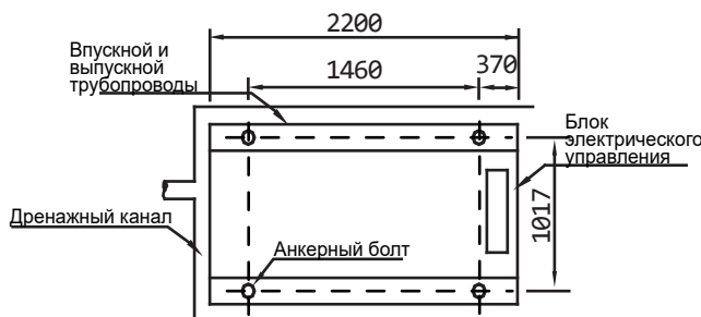
Схема монтажного основания для моделей MDVM-V90D2BR8-A - MDVM-V1402BR8-A
