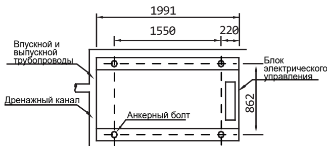
Схема монтажного основания для модели MDVM-V75D2BR8-A
