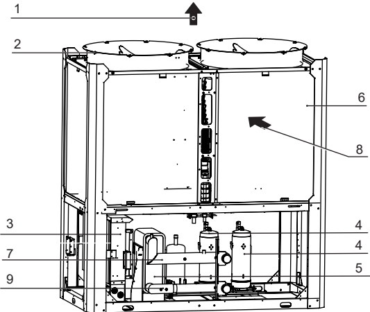
Модель MDVM-V140D2BR8-A
