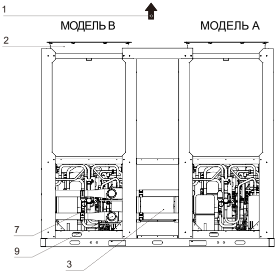
Модель MDVM-V180D2BR8-A
