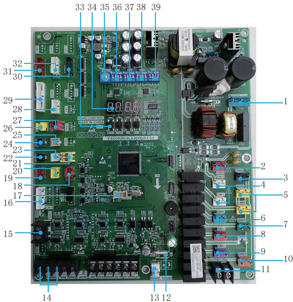
Плата управления ведущего чиллера для моделей MDVM-V75D2BR8-A и MDVM-140D2BR8-A
