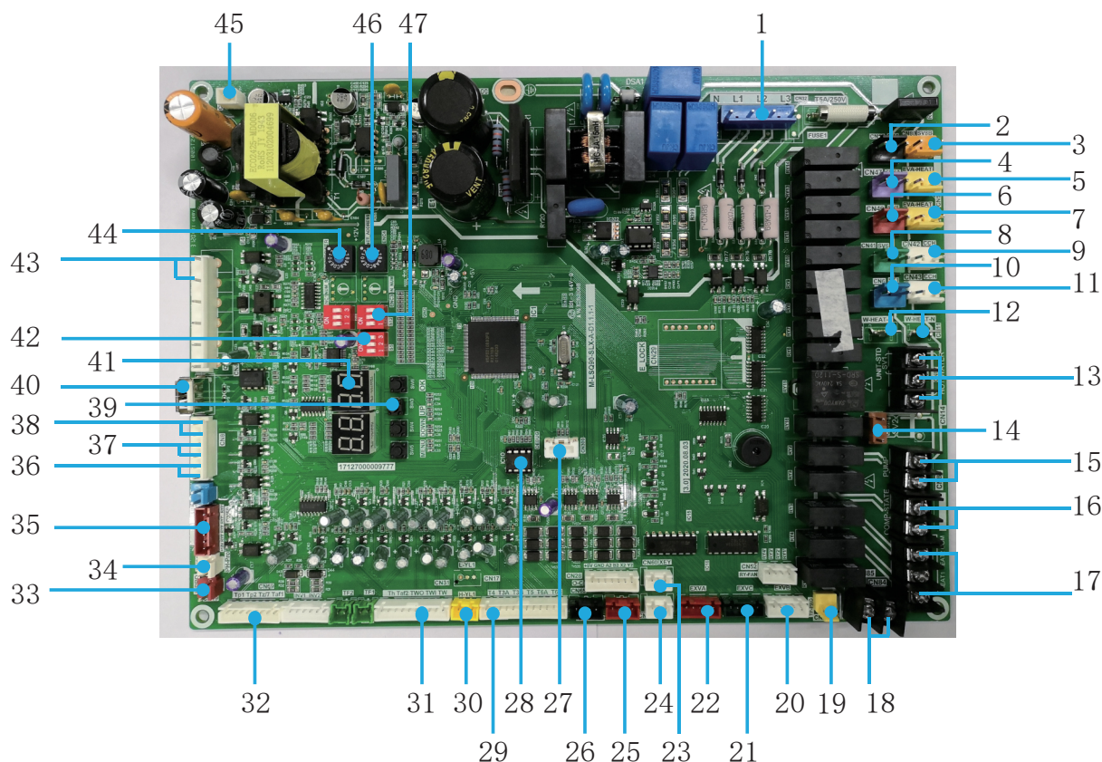
Плата управления ведущего чиллера для моделей MDVM-V90D2BR8-A и MDVM-180D2BR8-A
