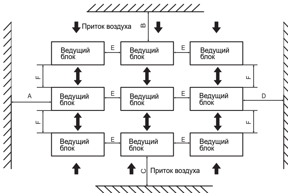
Монтаж модульной системы
