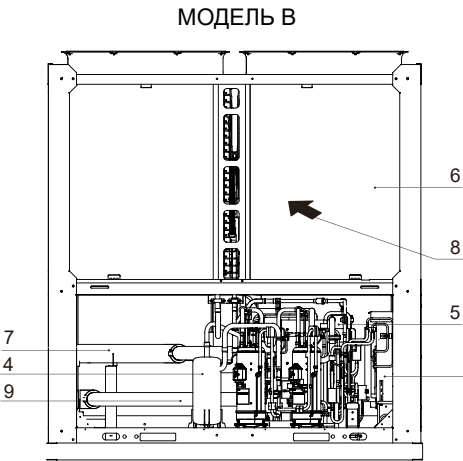
Модель MDVM-V180D2BR8-A
