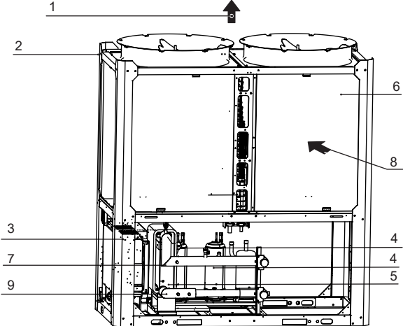
Модель MDVM-V90D2BR8-A
