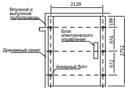
Схема монтажного основания для модели MDVM-V180D2BR8-A
