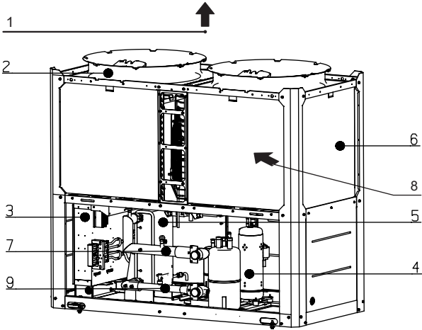
Модель MDVM-V75D2BR8-A
