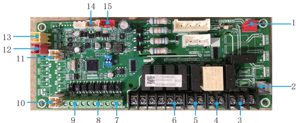
Плата управления ведомого чиллера для моделей MDVM-V75D2BR8-A и MDVM-140D2BR8-A
