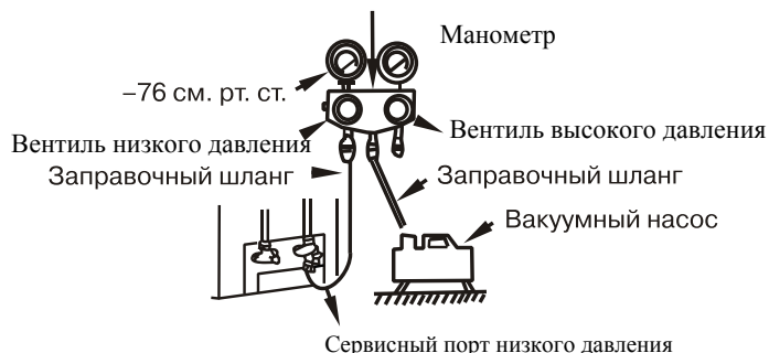
Манометрический коллектор
